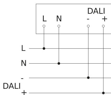
Schéma du circuit principal
